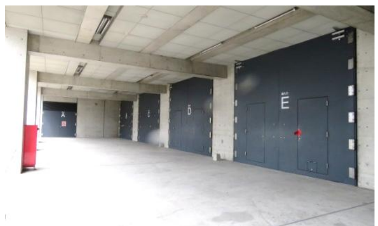
搬入口 幅 4.5m×高さ 3.9m
